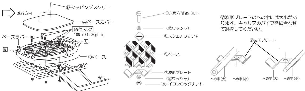
図 G（ベース取り付け概要図）
