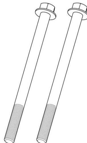
⑤フランジボルト (M10×145 / P1.25)
