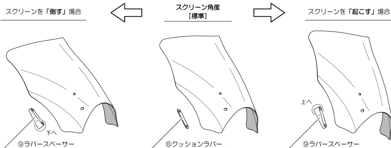
図5 ◇スクリーンの角度調整の方法と部品の選択
