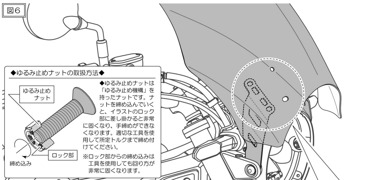
スクリーン角度「標準」の取付イメージ
