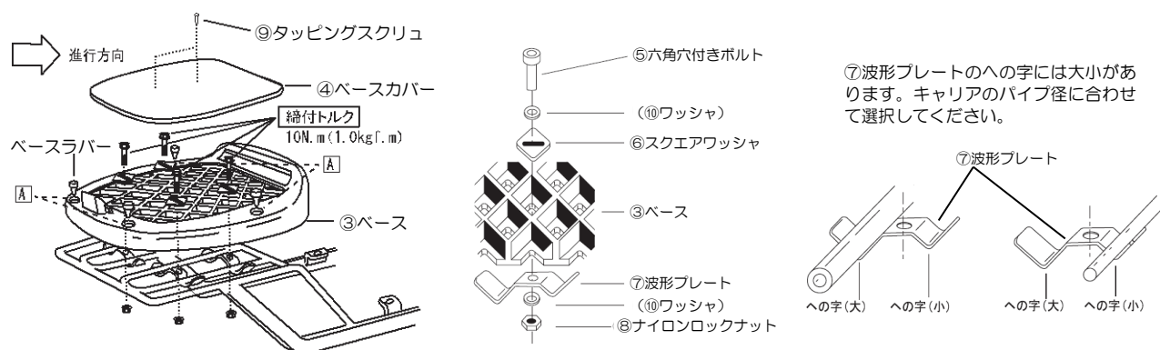
図 C（ベース取り付け概要図）
