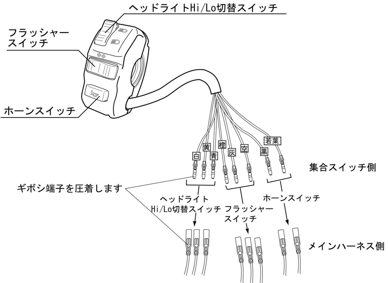
ヘッドライトHi/Lo切替スイッチ
