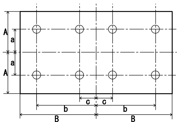
図 試験板
