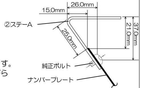
イラスト:寸法確認図
