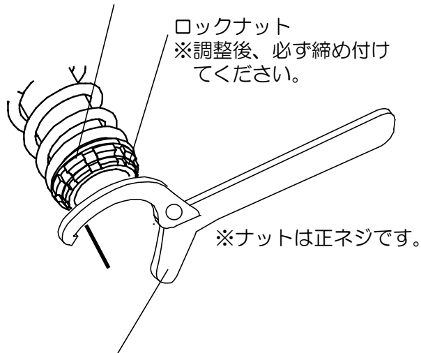
イニシャル調整ナット
