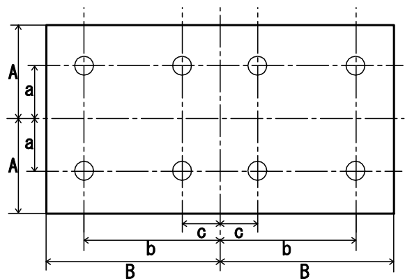
図 試験板
