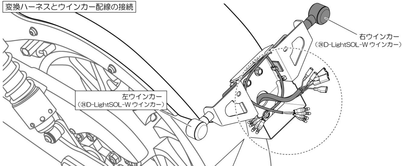
変換ハーネスとウィンカーの接続イラスト
