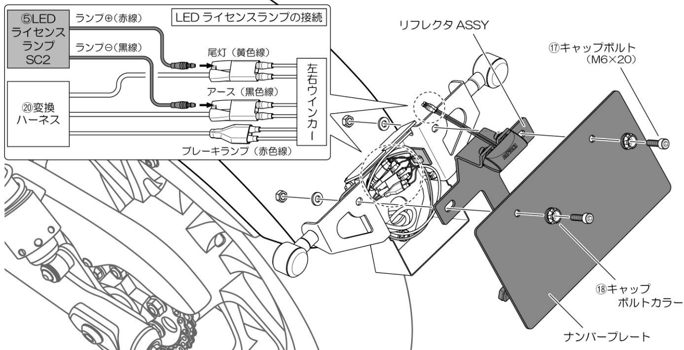
リフレクタ ASSYとナンバープレートの取り付け
