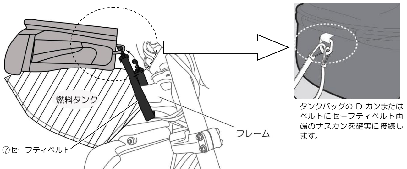
図 C: セーフティベルトを車両に固定
